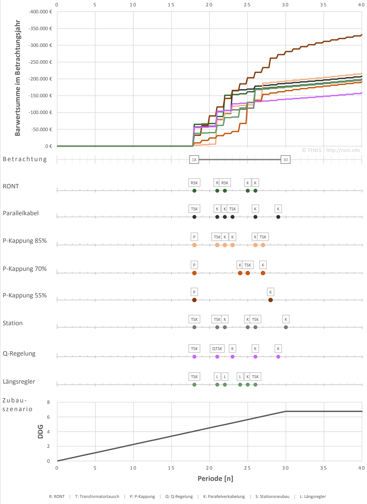
Abbildung 1: Zubau über 40 Jahre auf DDG_{norm} = 75\% , Stranganfang, i = 5\% | r = 1,5\% (KVE2)
