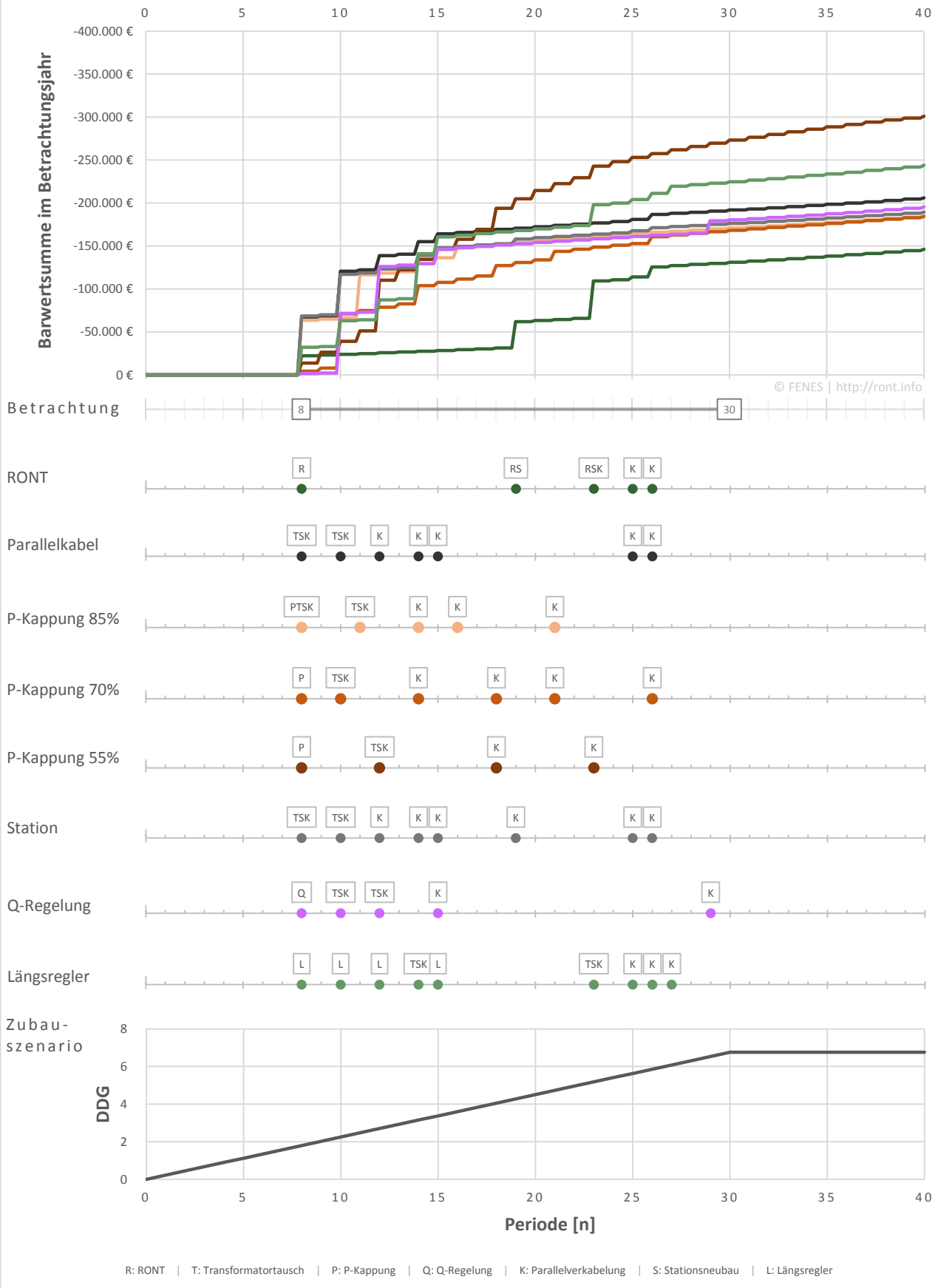
Abbildung 2: Zubau über 40 Jahre auf DDG_{norm} = 75\% , Strangende, i = 5\% \quad | \quad r = 1,5\% (KVE2)
