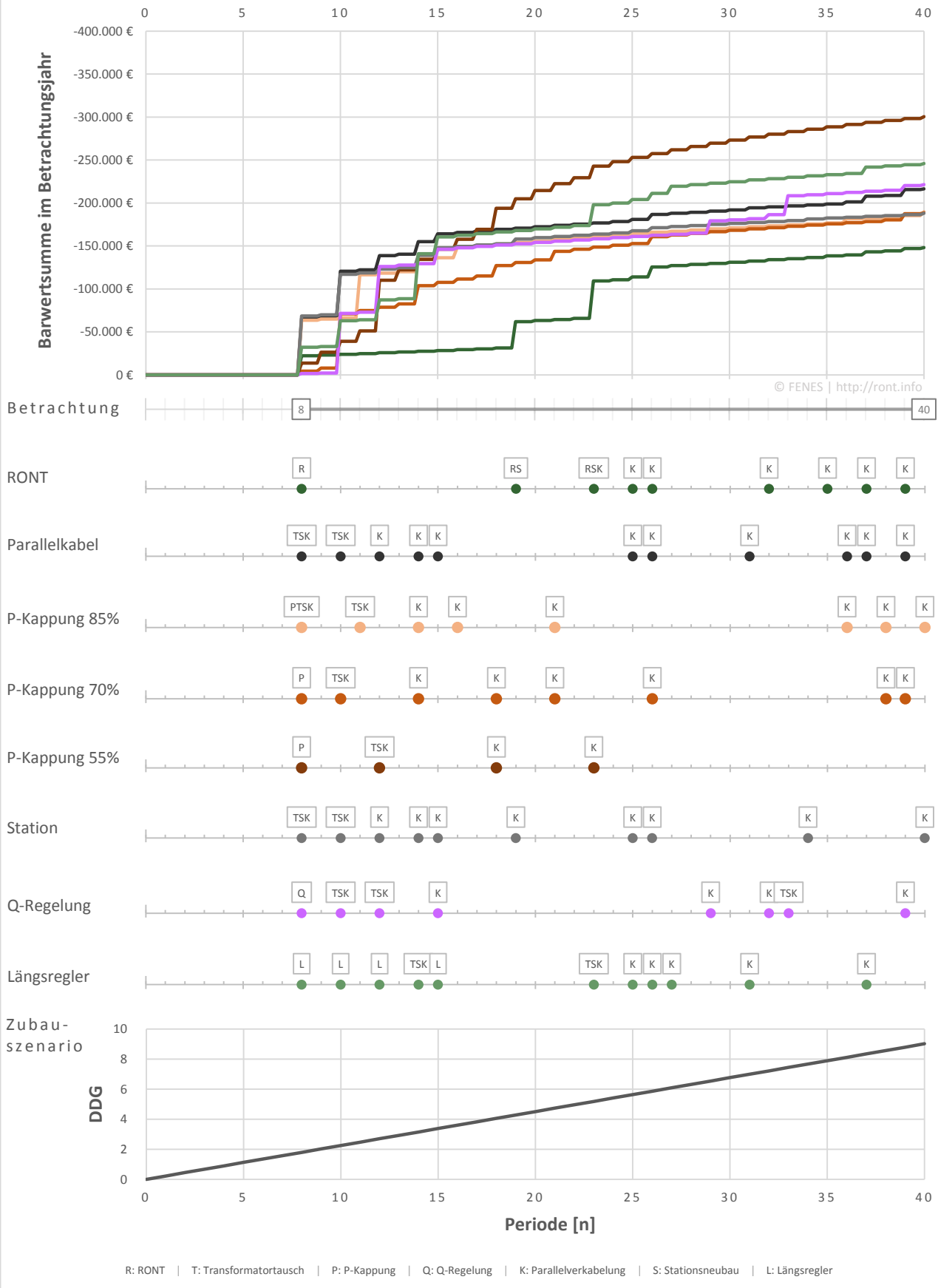
Abbildung 4: Zubau über 40 Jahre auf DDG_{norm} = 100\% , Strangende, i = 5\% | r = 1,5\% (KVE2)
