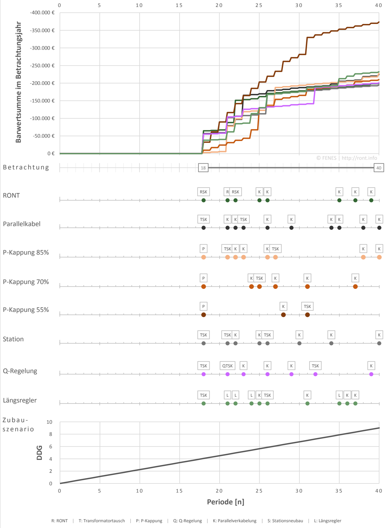
Abbildung 3: Zubau über 40 Jahre auf DDG_{norm} = 100\% , Stranganfang, i = 5\% | r = 1,5\% (KVE2)
