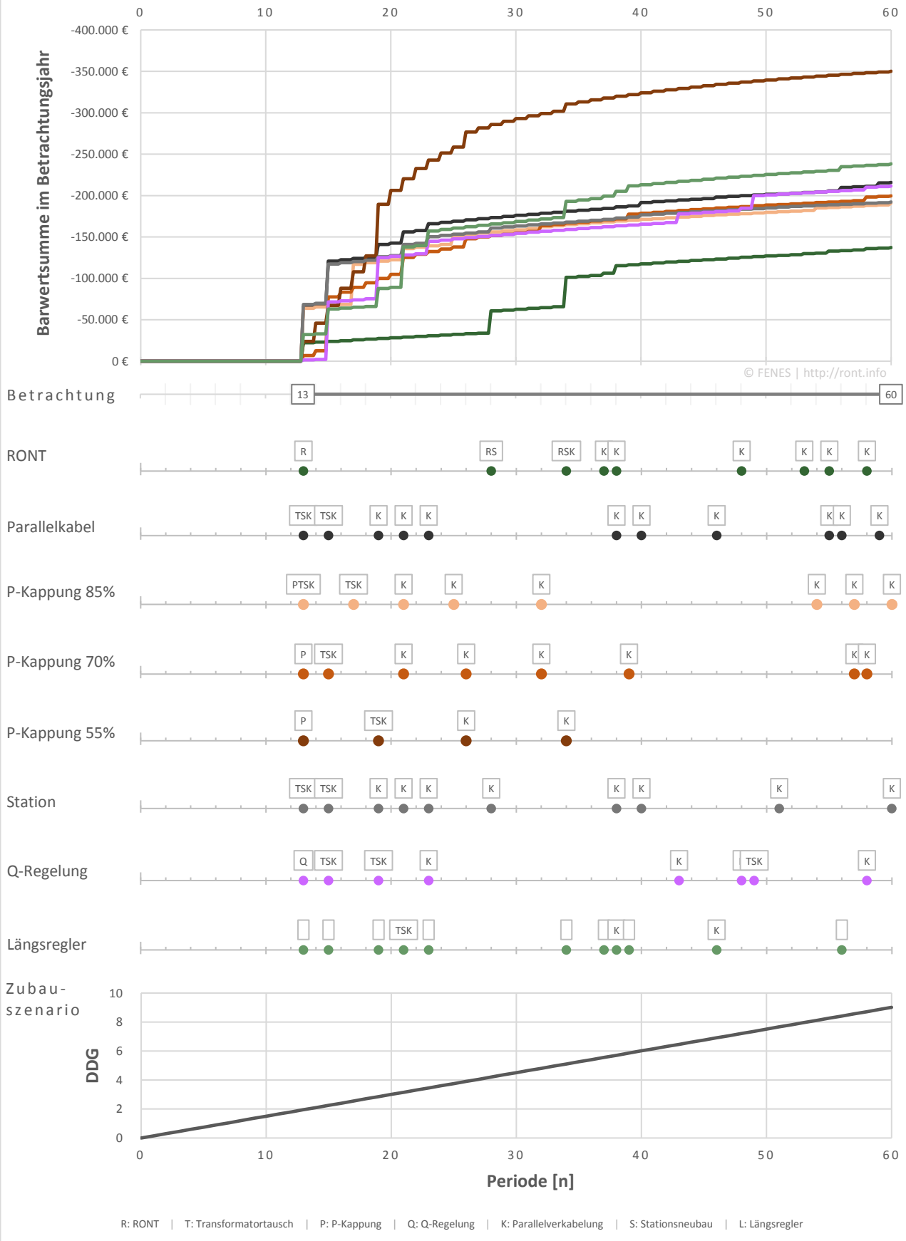
Abbildung 6: Zubau über 40 Jahre auf DDG_{norm} = 100\% , Strangende, i = 5\% | r = 1,5\% (KVE2)
